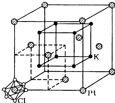
Рис. 3.108. Элементарная ячейка \text{K}_2[\text{PtCl}_6]
