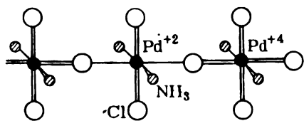
Рис. 3.111. Структура \text{PdCl}_3 \cdot 2\text{NH}_3
