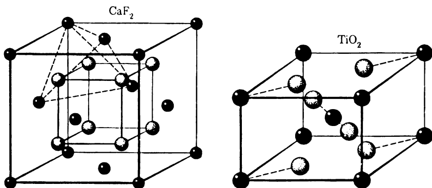
Рис. 1.81. Кристаллические решетки флюорита \text{CaF}_2 и рутила \text{TiO}_2 . Светлые шары – ионы \text{F}^- или атомы O, темные шары – ионы \text{Ca}^{2+} или атомы Ti
