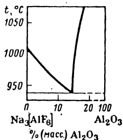
Рис. 3.9. Фрагмент диаграммы состояния системы \text{Na}_3[\text{AlF}_6]\text{--Al}_2\text{O}_3
