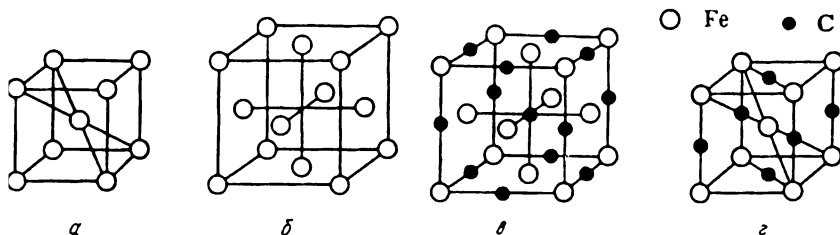
Рис. 3.98. Кристаллические структуры \alpha -Fe (а), \gamma -Fe (б), аустенита (в), мартенсита (г)
