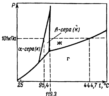
Рис. 3.48. Диаграмма состояния серы
