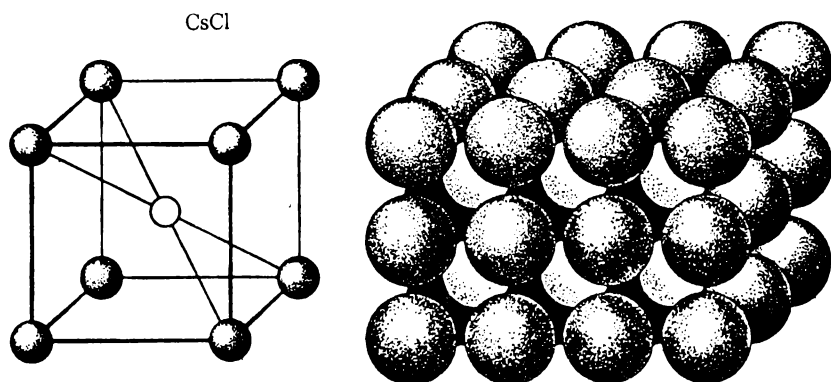
Рис. 1.76. Кристаллическая решетка хлорида цезия. Светлые шары – ионы \text{Cs}^+ , темные – ионы \text{Cl}^- . Слева показана ячейка CsCl
