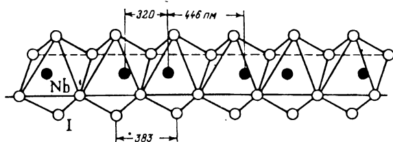
Рис. 3.80. Структура кристаллического NbI 4
