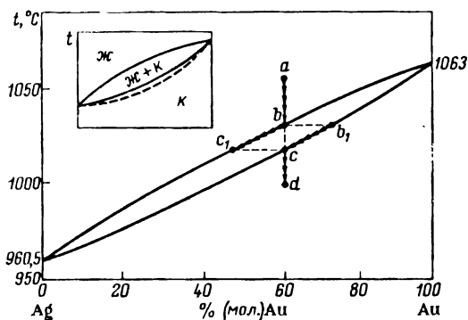
Рис. 2.35. Диаграмма состояния системы веществ, образующих твердые растворы.
