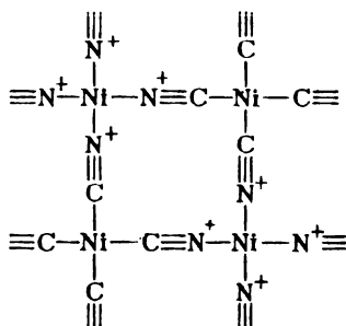
Рис. 3.106. Слой атомов в кристаллической решетке \text{Ni}(\text{CN})_2
