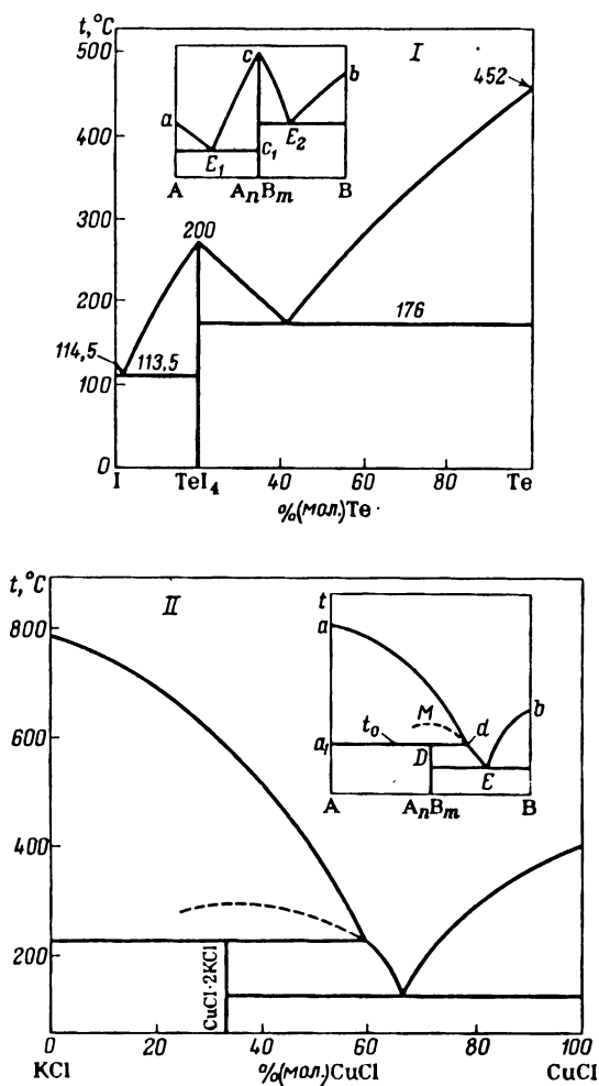
Рис. 2.34. Диаграмма состояния системы веществ, образующих устойчивое (вариант I) и неустойчивое (вариант II) химическое соединение A_nB_m . Примеры систем: I – Te с образованием \text{TeI}_4 (I); KCl – CuCl с образованием \text{K}_2\text{CuCl}_3 (II)
