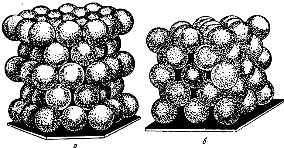
Рис. 1.75. Плотнейшие упаковки шаров: а – гексагональная; б – кубическая гранецентрированная
