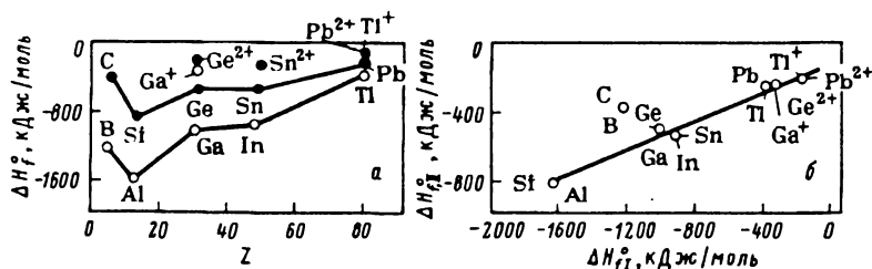
Рис. 3.28. Зависимость стандартных теплот образования оксидов элементов подгрупп IIIA и IVA от порядкового номера элемента (а) и взаимосвязь между стандартными теплотами образования оксидов элементов подгрупп IIIA и IVA (б)
