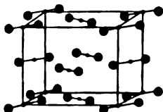
Рис. 3.59. Кристаллическая решетка иода
