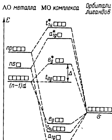
Рис. 1.60. Энергетическая диаграмма молекулярных орбиталей в октаэдрическом комплексе.
