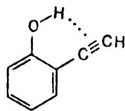
o-этинилфенол
