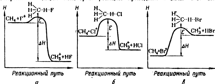
Рис. 2.15. Схема протекания процессов CH_4(r) + X^+(r) \longrightarrow CH_3^+(r) + HX(r) ; X = F (а), Cl (б), Br (в)
