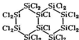
Рис. 3.33. Строение молекулы \text{Si}_{10}\text{Cl}_{18}
