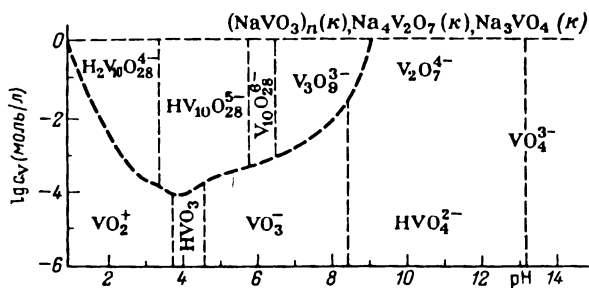
Рис. 3.81. Диаграмма состав раствора – pH для водных растворов ванадатов
