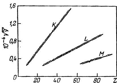
Рис. 1.14. Зависимость \sqrt{\tilde{\nu}} для линий серий K , L , M рентгеновского спектра от порядкового номера элемента
