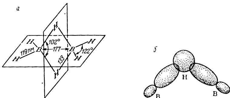
Рис. 1.52. Строение молекулы диборана B_2H_6 (а) и схема образования связей В—Н—В (б)
