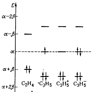
Рис. 1.49. Энергетические уровни \pi -электронов в молекуле этилена, радикале \cdot\text{C}_3\text{H}_5 и образованных из него ионах
