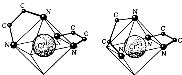
Рис. 1.54. Пространственные структуры оптических изомеров комплексов хрома с этилендиамином.
