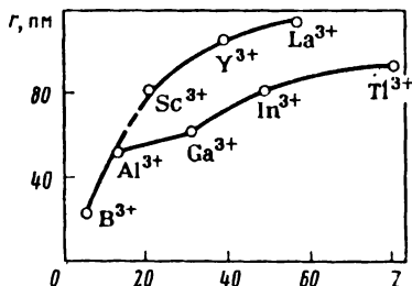
Рис. 3.11. Зависимость радиусов ионов элементов III группы от порядкового номера элемента
