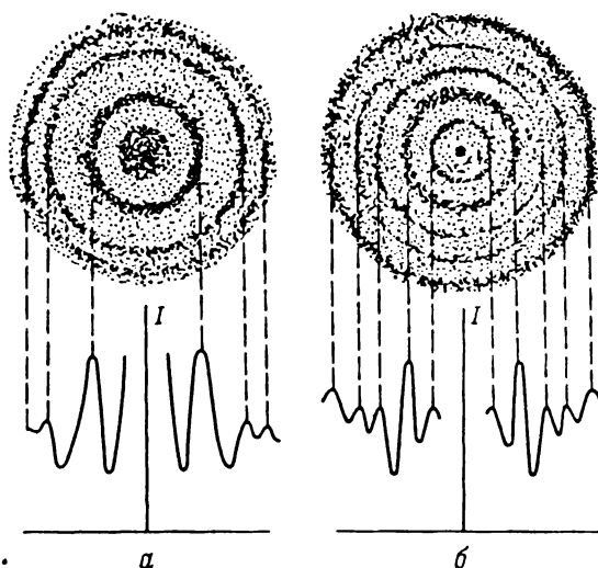
Рис. 1.24. Электрограммы \text{CCl}_4 (а) и \text{CS}_2 (б).
