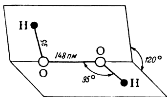
Рис. 3.47. Строение молекулы \text{H}_2\text{O}_2
