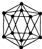
Рис. 3.8. Структура кристаллического бора Решетка состоит из икосаэдров [B_{12}] , к.ч. 5, d(B-B) = 194 пм
