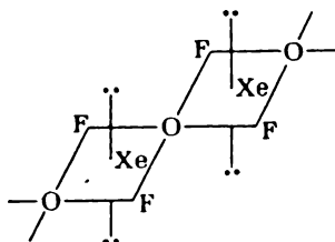
Рис. 3.63. Кристаллическая решетка \text{XeF}_2
