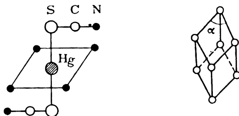
Рис. 3.120. Элементарная ячейка кристаллической решетки ртути ( \alpha = 70^\circ 32' ).
