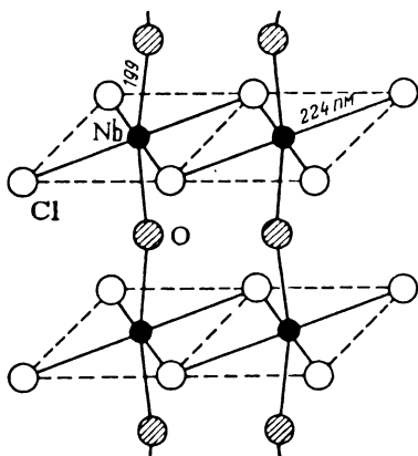
Рис. 3.84. Структура кристаллического оксохлорида \text{NbOCl}_3
