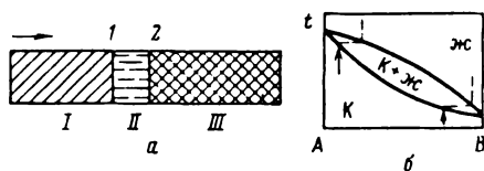
Рис. 3.26. Схема процесса зонной очистки (а) и диаграмма состояния системы с непрерывным рядом твердых растворов (б):
