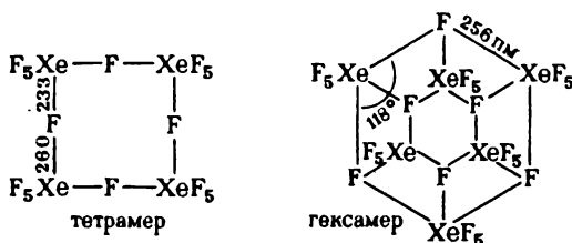
Рис. 3.65. Фрагменты структуры \text{XeF}_6(\kappa)
