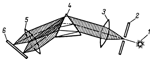
Рис. 1.1. Схема действия спектрографа:
