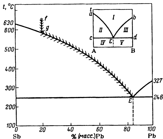
Рис. 2.33. Диаграмма состояния системы веществ (Sb-Pb), образующих эвтектическую смесь
