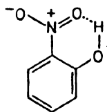
o-нитрофенол
