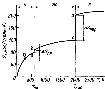
Рис. 2.5. Зависимость энтропии свинца от температуры:
