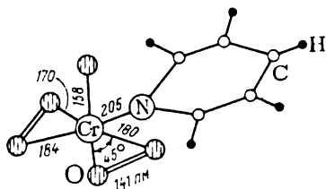
Рис. 3.92. Строение молекулы \text{CrO}_5 \cdot \text{C}_5\text{H}_5\text{N}
