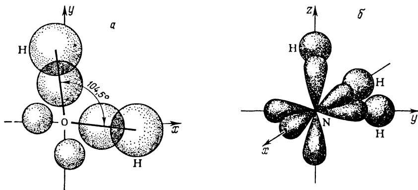
Рис. 1.34. Перекрывание атомных орбиталей при образовании молекул \text{H}_2\text{O} (а) и \text{NH}_3 (б)
