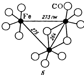
Рис. 3.101. Строение молекулы карбонилы [\text{Co}_2(\text{CO})_8] (а) и [\text{Fe}_3(\text{CO})_{12}] (б)
