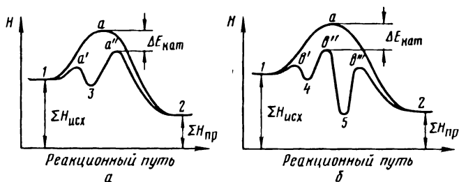
Рис. 2.16. Влияние катализатора на протекание реакции при гомогенном (а) и гетерогенном (б) катализе:
