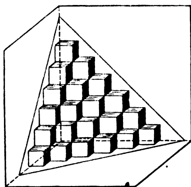
Рис. 1.67. Иллюстрация закона целых чисел:
