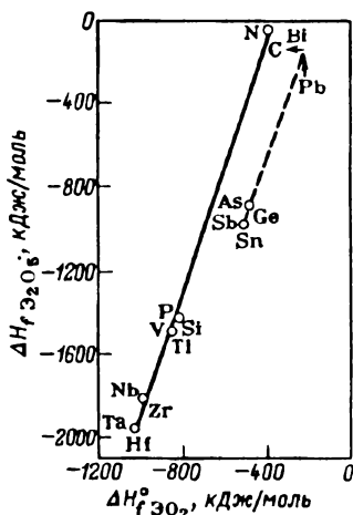
Рис. 3.71. Взаимосвязь между стандартными энтальпиями образования высших оксидов элементов IV и V групп
