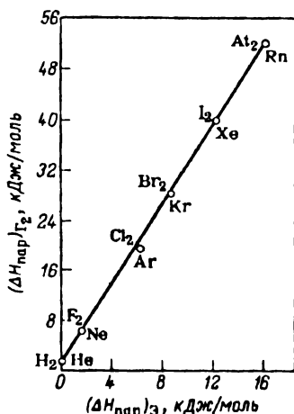
Рис. 3.62. Взаимосвязь между теплотами парообразования элементарных веществ подгрупп VIII A (3) и VIII A (2)
