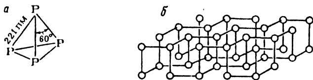
Рис. 3.42. Строение молекулы P_4 (а) и кристаллическая решетка черного фосфора (б)
