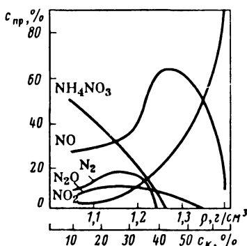
Рис. 3.41. Зависимость содержания спир различных продуктов восстановления железом \text{HNO}_3 от ее плотности \rho (концентрации c_k )
