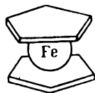
Рис. 3.104. Структура ферроцена (схема)
