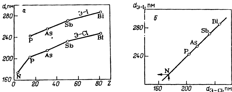
Рис. 1.15. К определению межатомного расстояния в молекулах методом сравнительного расчета:
