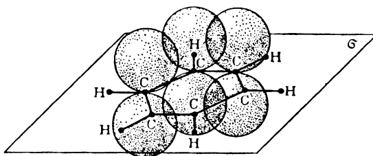
Рис. 1.43. Схема образования химических связей в молекуле C_6H_6 . Чтобы не загромождать чертеж, показаны только три p -орбитали
