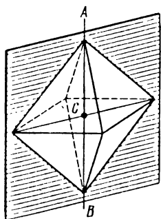
Рис. 1.69. Элементы симметрии октаэдра: центр симметрии C , ось симметрии AB ( n=4 ), плоскость симметрии (заштрихована).
