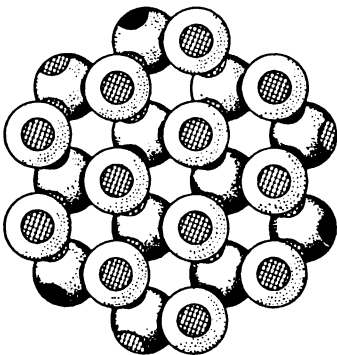
Рис. 1.80. Структура льда
