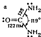
Рис. 3.31. Строение молекулы карбамида (а) и тиокарбамида (б)
