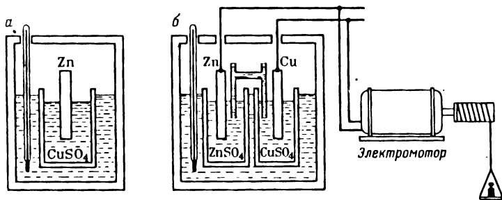
Рис. 2.9. Варианты проведения реакции \text{Zn (к)} + \text{CuSO}_4(\text{р}) \longrightarrow \text{Cu (к)} + \text{ZnSO}_4(\text{р}) при 25 °С и 101 кПа:
