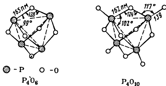
Рис. 3.44. Строение молекул P_4O_6 и P_4O_{10}
