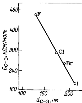
Рис. 1.22. Взаимосвязь энергий и длин связи в молекулах галогенидов углерода
