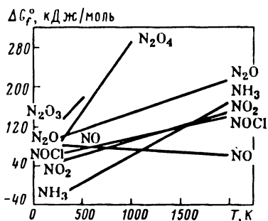
Рис. 3.40. Зависимость изменения стандартной энергии Гиббса образования некоторых соединений азота от температуры
