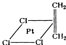
Рис. 1.62. Строение иона [\text{Pt}(\text{C}_2\text{H}_4)\text{Cl}_3]^-
