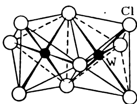
Рис. 3.88. Структура аниона (W_2Cl_6)^{3-}
