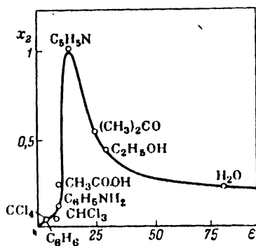
Рис. 2.19. Зависимость растворимости резорцина от диэлектрической проницаемости растворителя при 30° С
