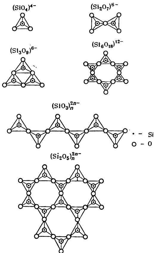
Рис. 3.24. Строение анионов кремниевых кислот
