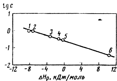
Рис. 2.18. Взаимосвязь между теплотой растворения \Delta H_p и растворимостью газов с в \text{C}_2\text{H}_5\text{OH} при 25^\circ\text{C} : 1 — He; 2 — Ne; 3 — \text{N}_2 ; 4 — CO; 5 — Ar; 6 — \text{CO}_2
