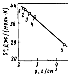
Рис. 3.23. Взаимосвязь между плотностью различных модификаций \text{SiO}_2 и их энтропией:
